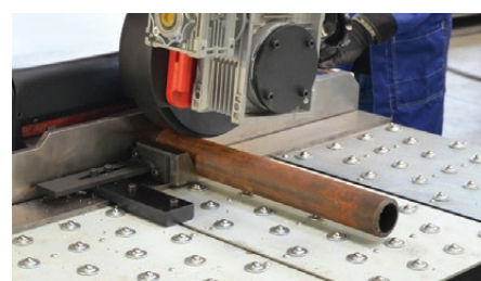
Possibility of pipe OD beveling
